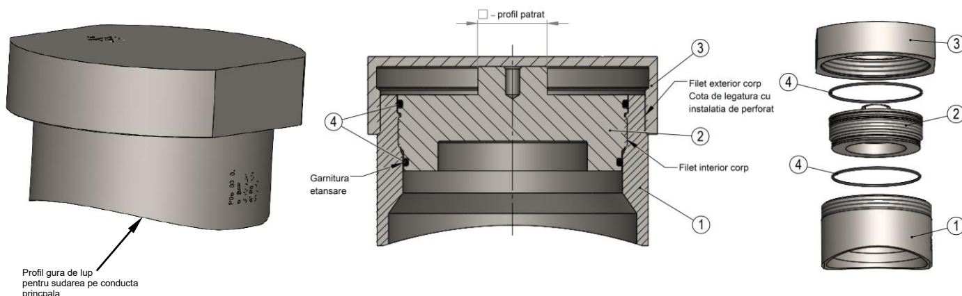
Fig. 1 Teu (picaj) pentru obturat conducte
