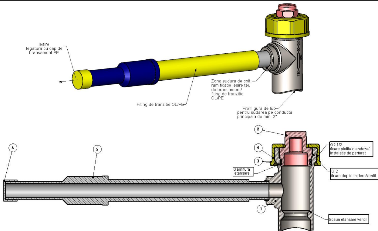
Fig. 1 Teu de bransament din otel cu dop si cu fitting de tranzitie OL/PE
