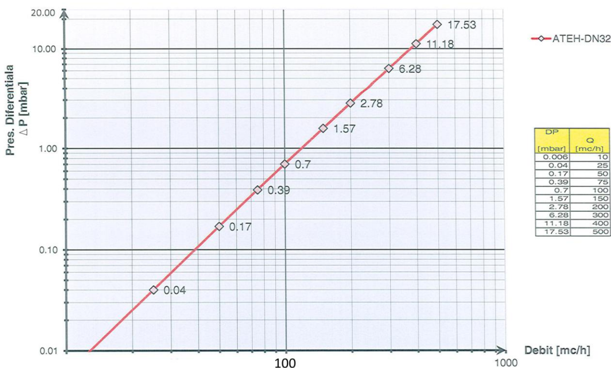
DIAGRAMA DE CALCUL CADERE DE PRESIUNE FUNCTIE DE DEBIT ATEH DN 32
